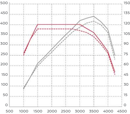
● : KOPPEL - ● : VERMOGEN STIPPELLEIJN EU6B (PH1) LIJN EU6DTEMP (PH2)
