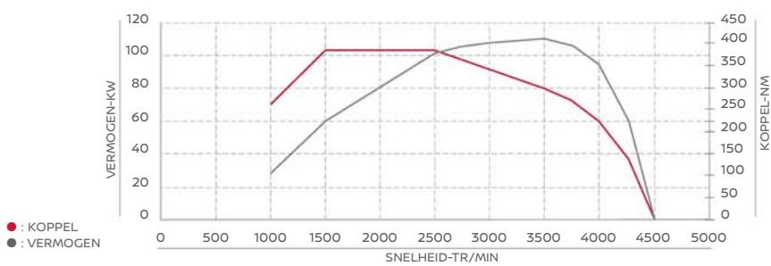
TECHNISCHE UITLEG: KOPPEL: 385 NM BIJ 1500 TPM VERMOGEN: 110 KW BIJ 3500 TPM
