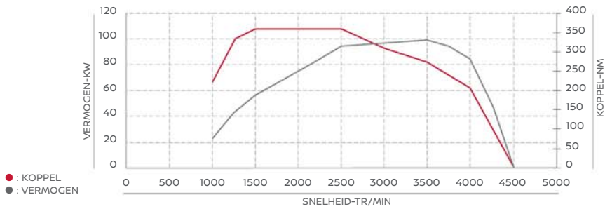
TECHNISCHE UITLEG: KOPPEL: 360 NM BIJ 1500 TPM VERMOGEN: 100 KW BIJ 3500 TPM
